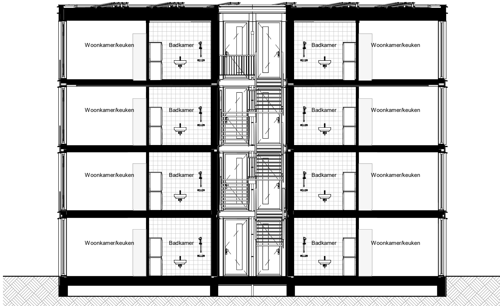
Doorsnede A
